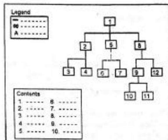
Fig. 4.6 HIPO diagram
